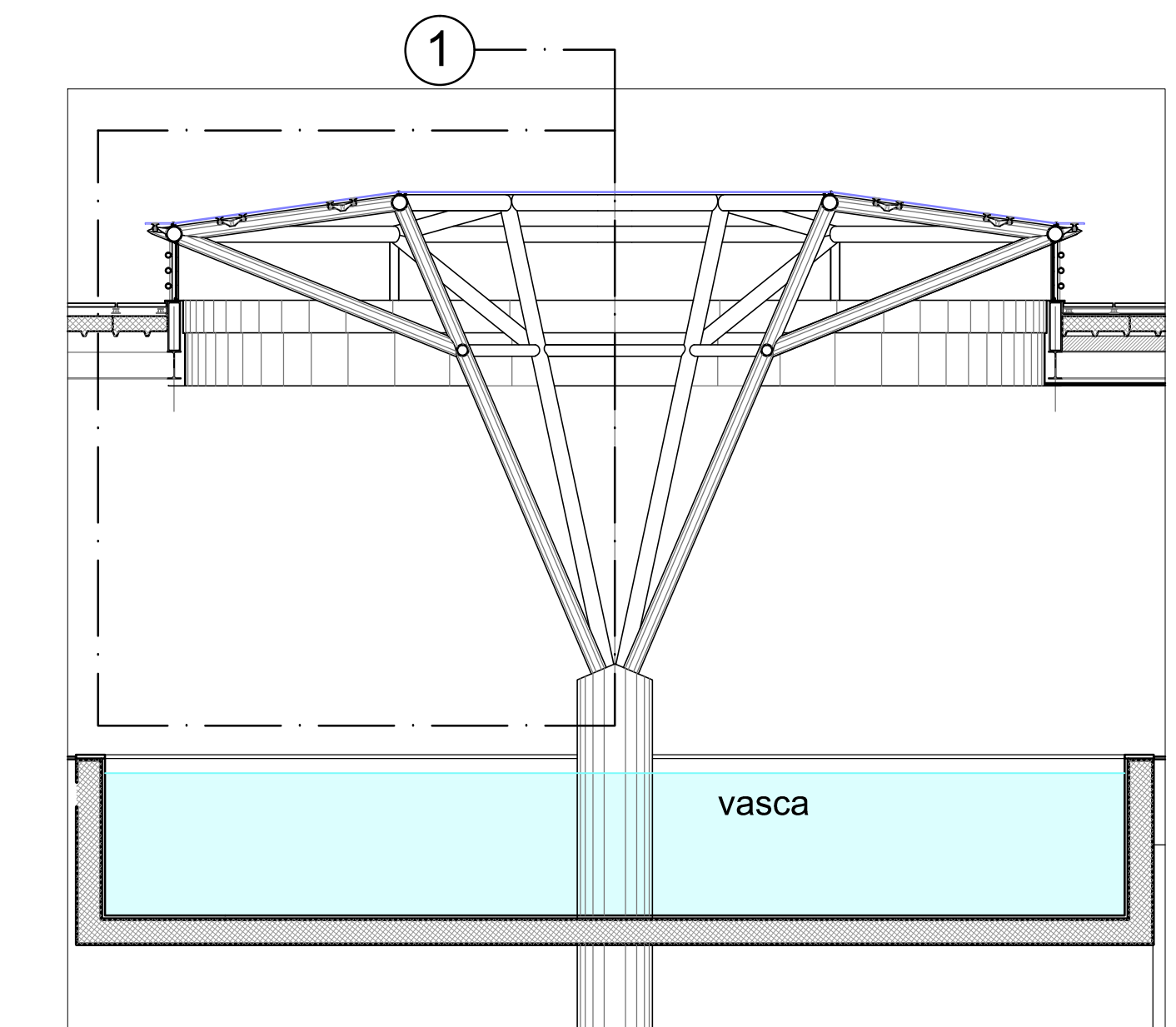
STRALCIO SEZIONE 4-4' 1:50
