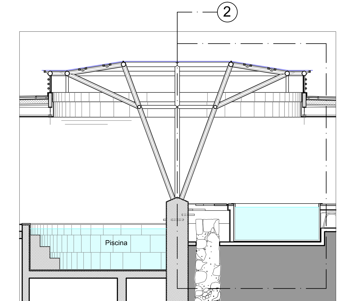
STRALCIO SEZIONE 7-7' 1:50
