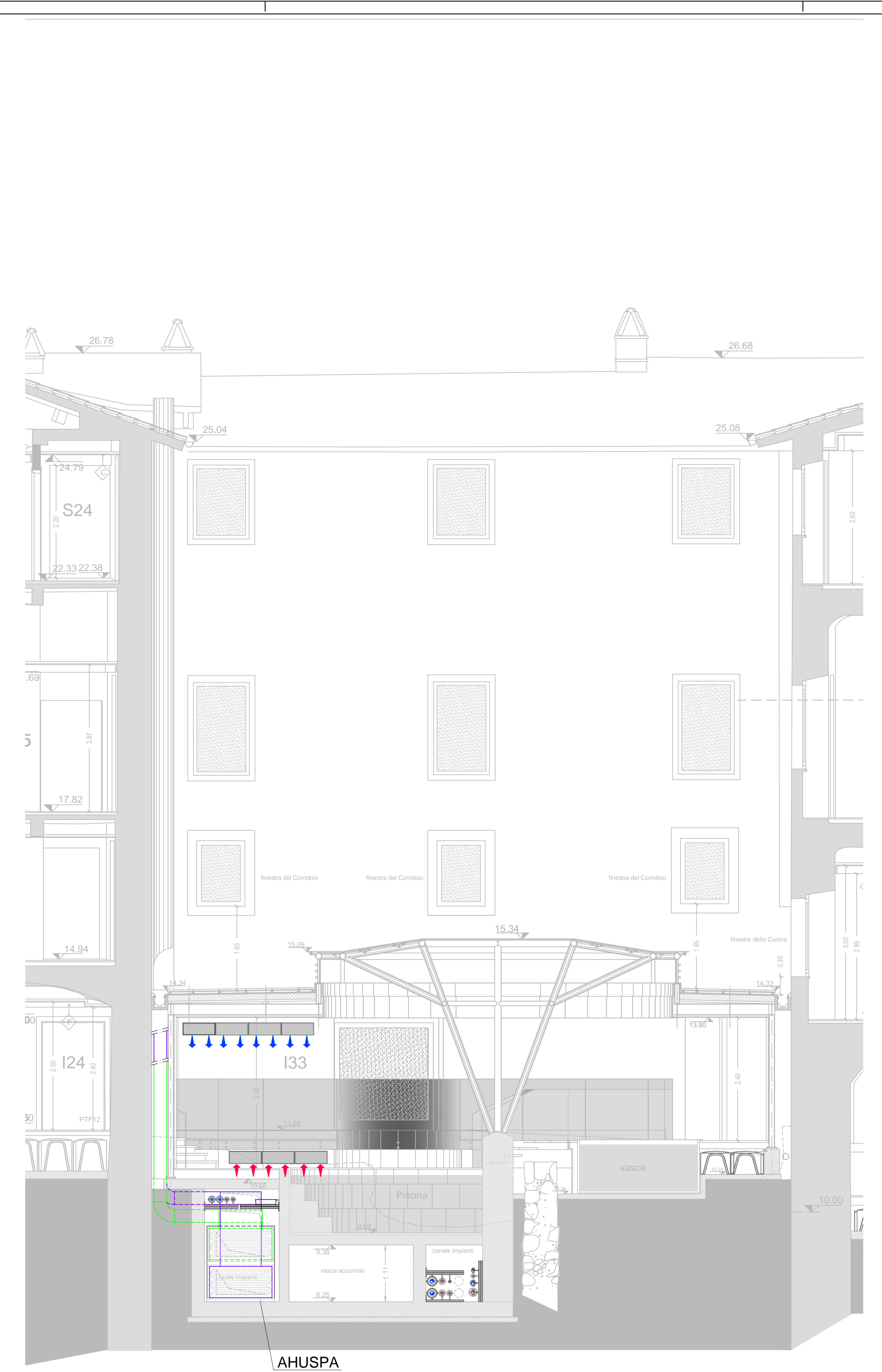
STRALCIO SEZIONE 7-7'
