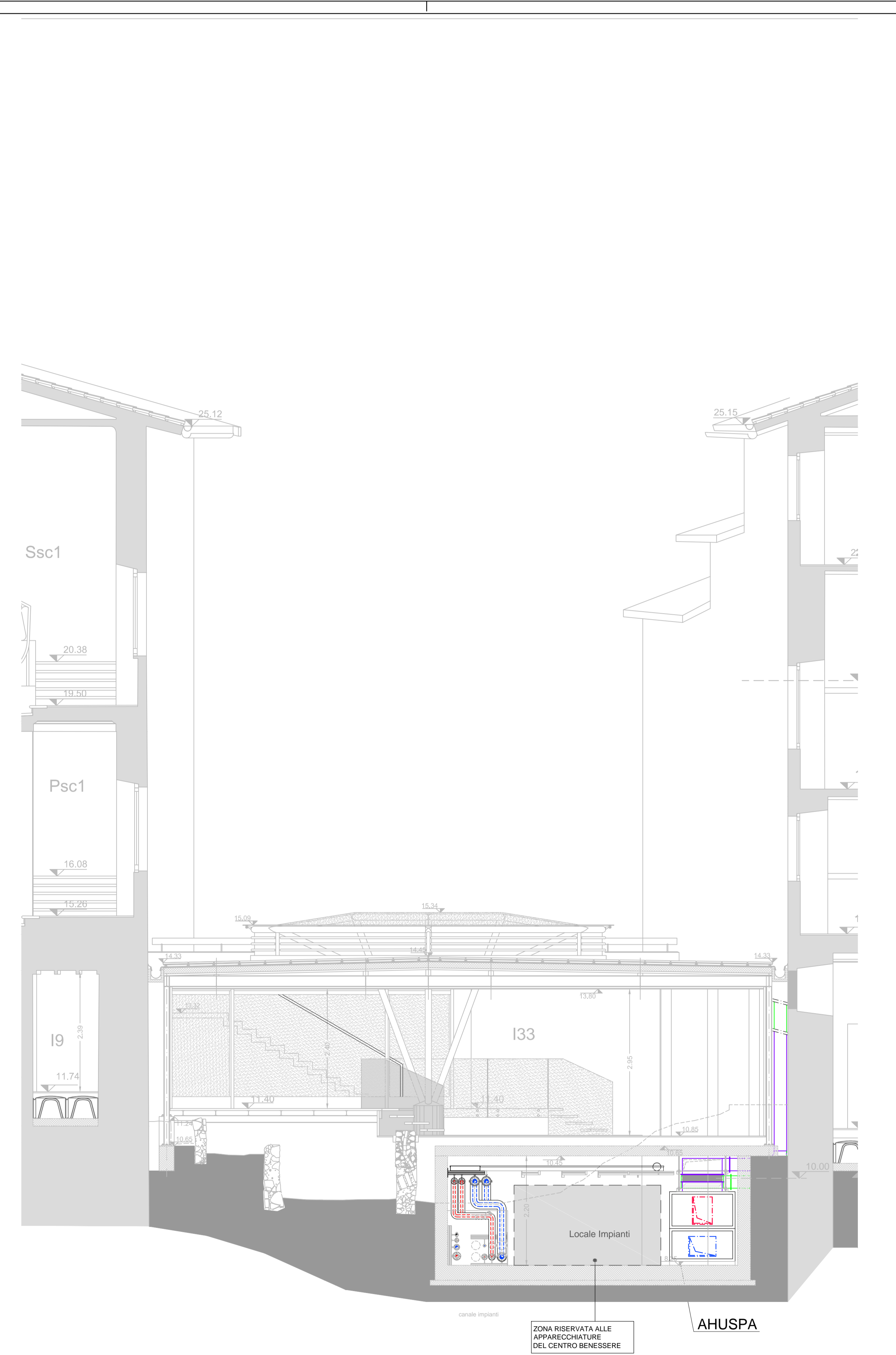
STRALCIO SEZIONE 8-8'
